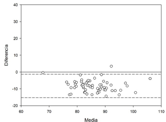
Figura 2. Gráficos de Bland-Altman para Glucosa
