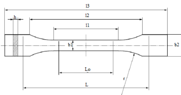
Figura 1. Molde de probeta Tipo B para plástico reforzado con fibra vegetal.
